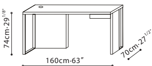
C05D1104+(C07D1107+C07D1108)
